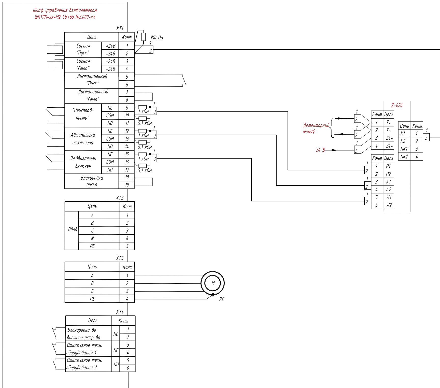
Схема подключения шкафа управления насосами ШК1101-XX-M2.
